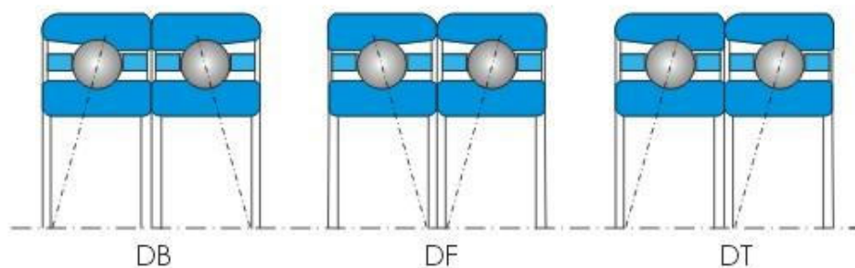
轴承双联配置形式 Duplex Pairings
