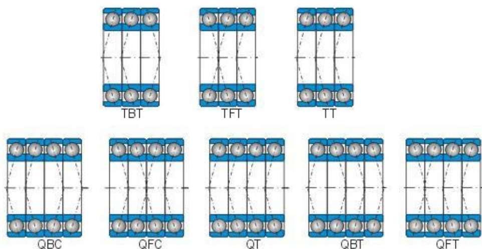
常用多联组配轴承的配置形式 Triplex and Quadruplex
